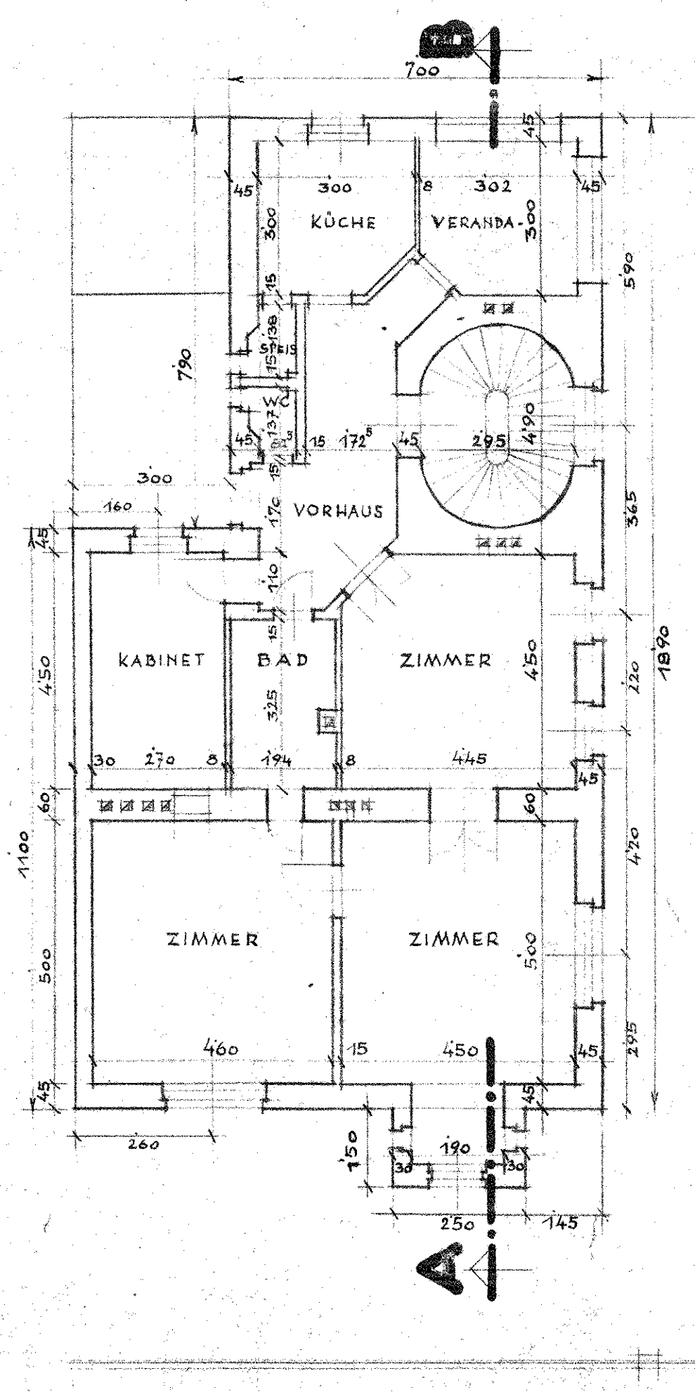
PARTERRE
