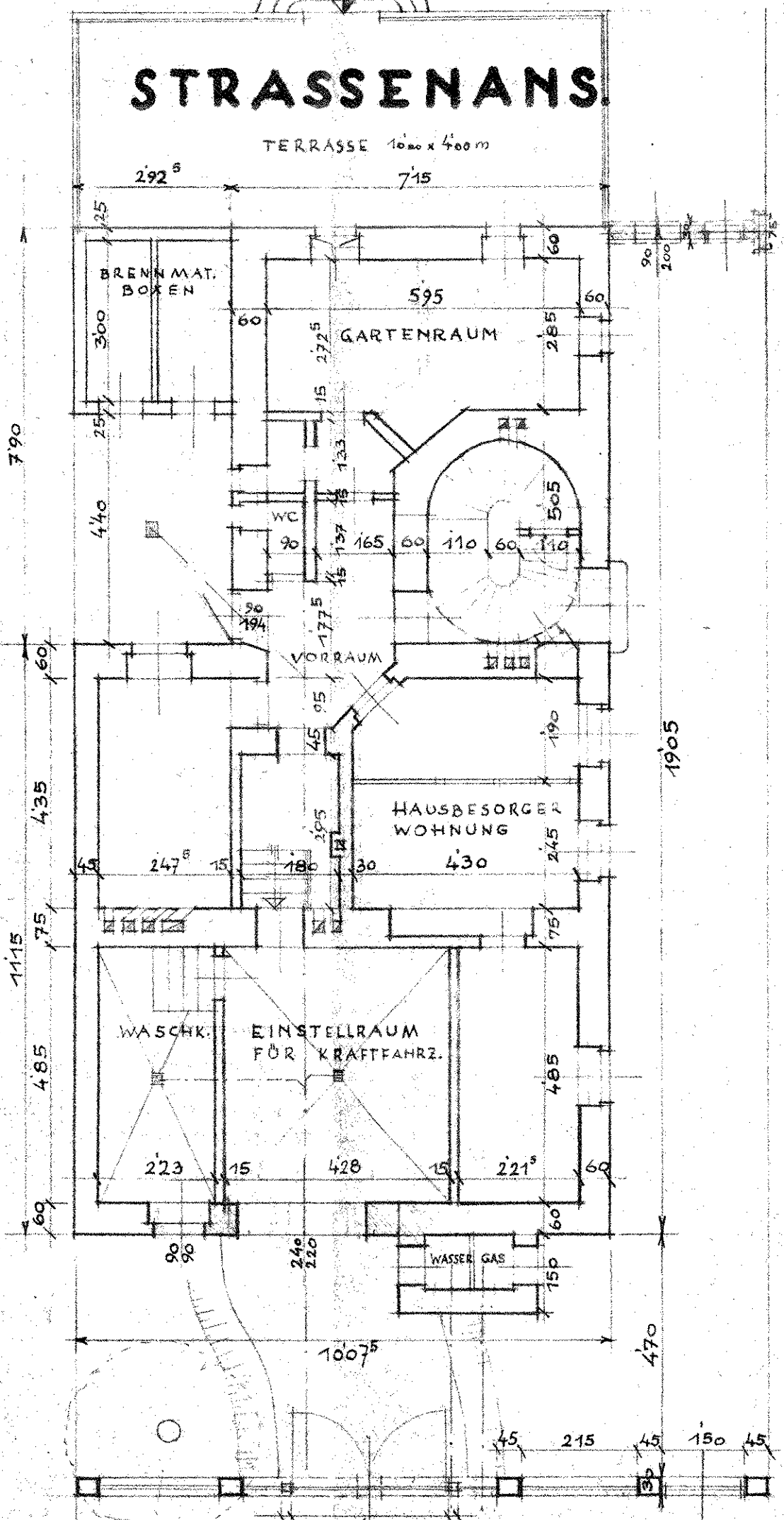
SOUTERRAIN
